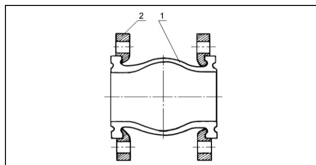
Рис. 7. Гибкая вставка типа ZKB. 1 – Гибкий элемент из армированной резины (EPDM или NBR); 2 – Фланец (2 шт.)
