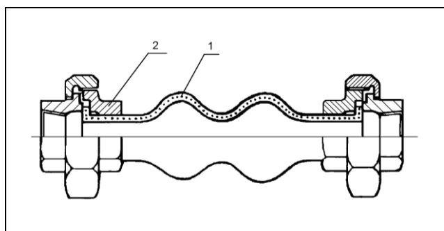
Рис. 6. Гибкая вставка типа ZKT 1 – Гибкий элемент из армированной резины (EPDM или NBR); 2 – Резьбовые соединительные элементы
